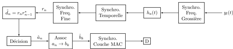
FIGURE 2 – Chaîne de réception incluant les blocs de synchronisations.
